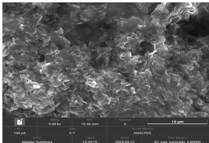
Figura 2. Foto da amostra SC com surfactante, não sonicada, filtrada em 0,8 µm (MEV).
