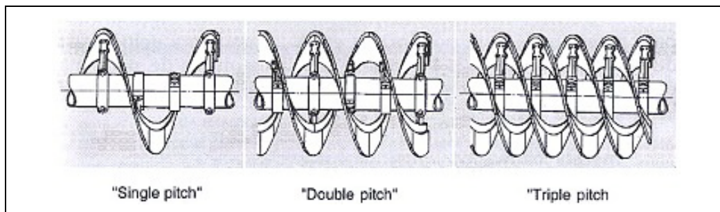
Figura 22 – Roscas simples, dupla e tripla.
