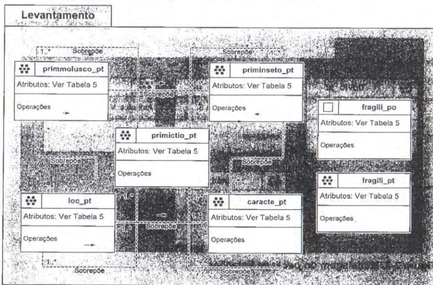
Figura 2-5. Modelagem do package Levantamento.
